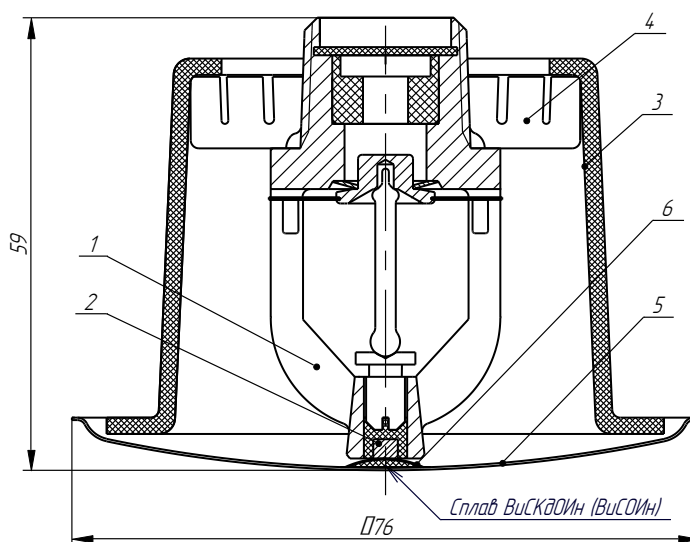
Рисунок 2 – Распылитель «РС-С»
